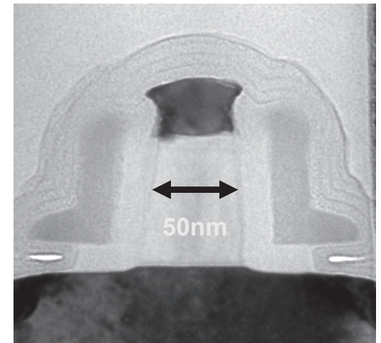
90nm MOS Transistor
