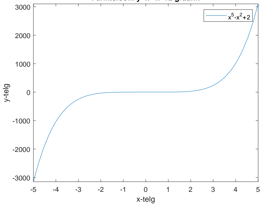
Funktsiooni y=x^5-x^2+2 graafik
