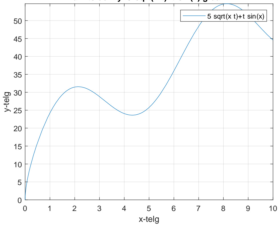
Funktsiooni y=5\sqrt{x*t}+t\sin(x) graafik
