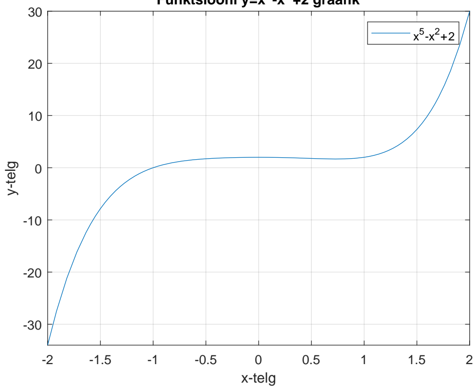
Funktsiooni y=x^5-x^2+2 graafik
