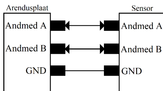
Joonis 6. RS-485 ühendus
